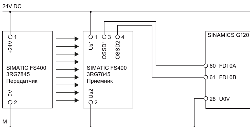
Изображение 5-44 Подключение электронного датчика в электрощкафу
