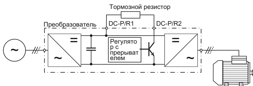
Изображение 5-11 Реостатное торможение с тормозным прерывателем в преобразователе
