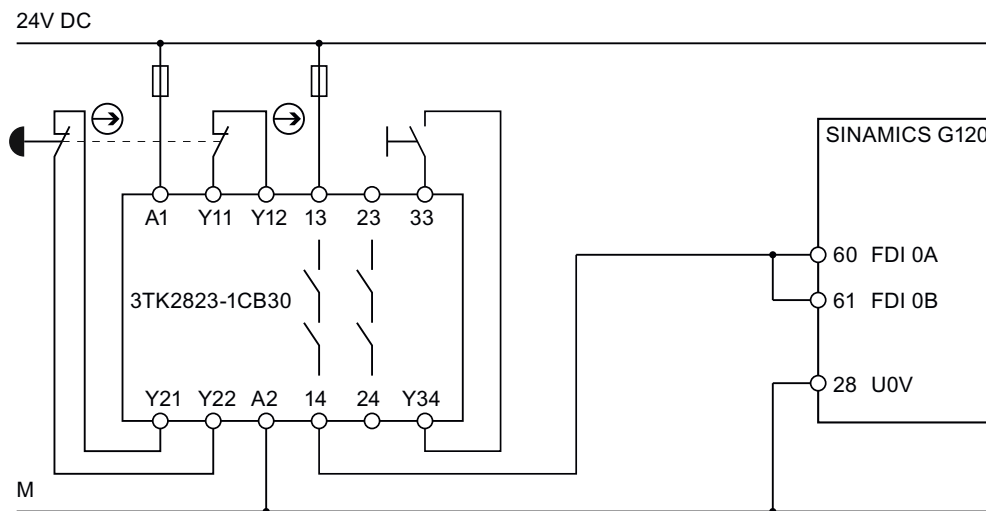
Изображение 5-45 Подключение устройства аварийной защиты в электрощкафу
